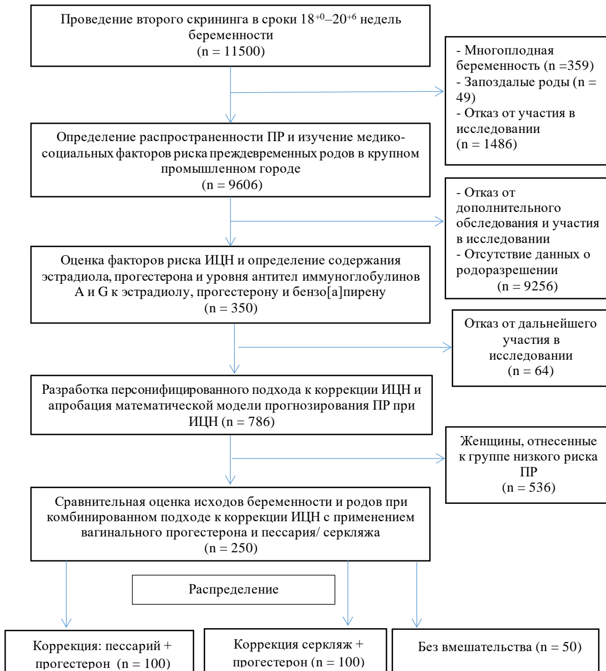
Рисунок 2 — Блок-схема исследования
